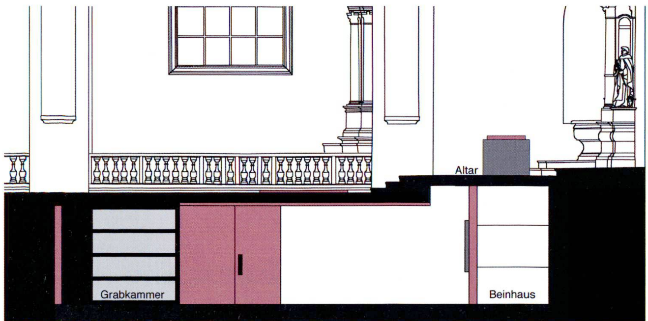
Längsschnitt Gruft
