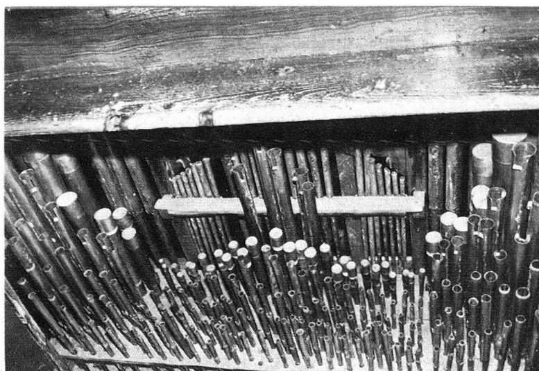
Abb. 9. Pfeifenanordnung im Rückpositiv der Orgel von Münster (vgl. Abb. 5). Im Hintergrund die Rückseiten der Prospektpfeifen
