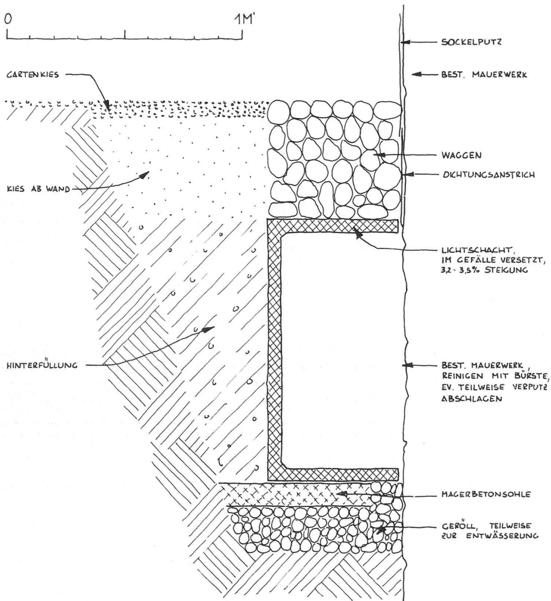
Abb. 1. Mauerbelüftung
