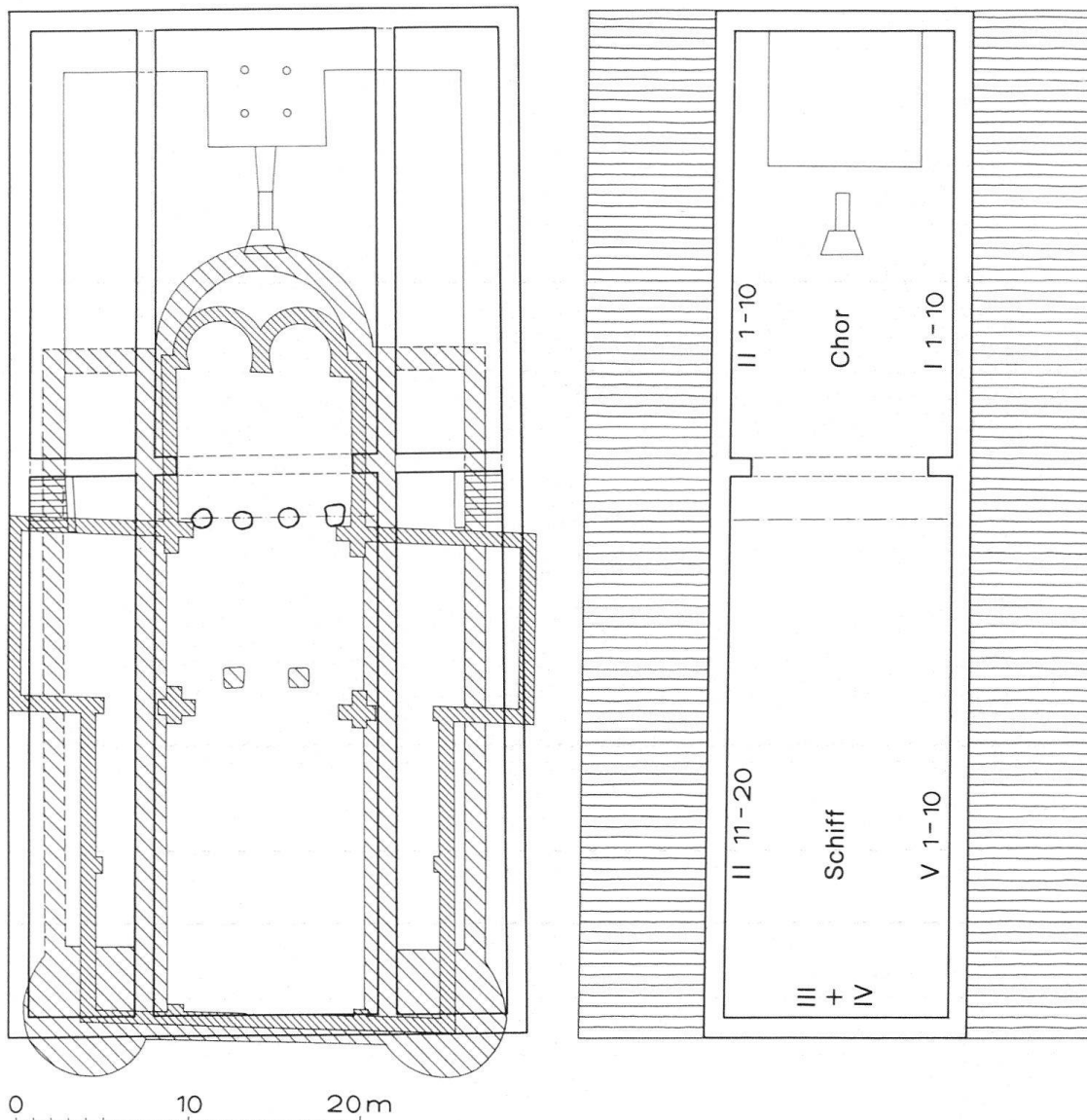
Abb. 2. St. Gallen, Das Münster des Abtes Gozbert im Verhältnis zu den Bauten Haitos. Weit schraffiert: Kathedrale Basel, eng schraffiert: Klosterkirche von Reichenau-Mittelzell Abb. 3. St. Gallen, Gozbertmünster, Grundriss des Obergadens. Anordnung der Wandgemälde nach den Tituli der Carmina Sangallensia
