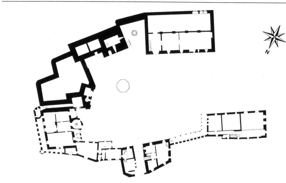
3 Grundriss von Dieter Boller, 1973 (Situation nach der Sanierung 1; von Einzelheiten abgesehen noch heute gültig).
