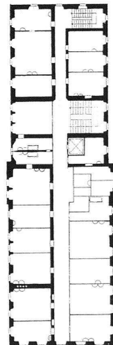
7 Zermatt, Hotel Mont Cervin, Grundriss-Aufnahme, 1943. – Gut sichtbar ist das etappenweise Anwachsen des Hotels aus einem kleinen Gebäude von 1852 (oben, mit Treppe), über die Erweiterung von 1856 (sieben Fensterachsen) zur Grundrissverdoppelung von 1875 (vgl. Abb. 3).
