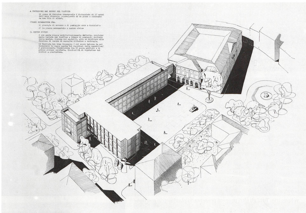
5 Secondo concorso bandito nel giugno 1949, motto 23.59.49, primo progetto acquistato, architetti Carlo e Rino Tami (Lugano), Vista assonometrica del complesso adibito ad uffici amministrativi dello Stato, Archivio del Moderno, Mendrisio.
