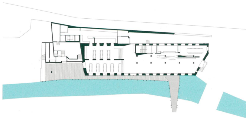
Grundriss Erdgeschoss
