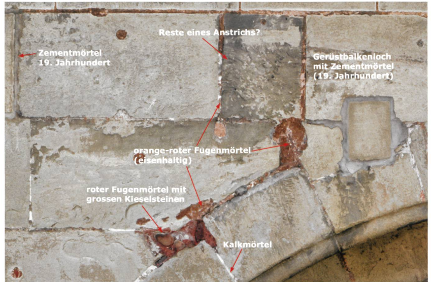
Von Ersatzmassnahmen verschont, ist das Obergadenfenster 90 an der Südseite des Chores eine bereichende Quelle der Baugeschichte. Der mittelalterliche Bestand zeigt Spuren verschiedener Restaurierungsphasen (unten: Gesamtansicht, oben: Detailausschnitt, 2016). © Berner Münster-Stiftung
