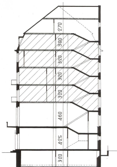
SCHNITT A-A
