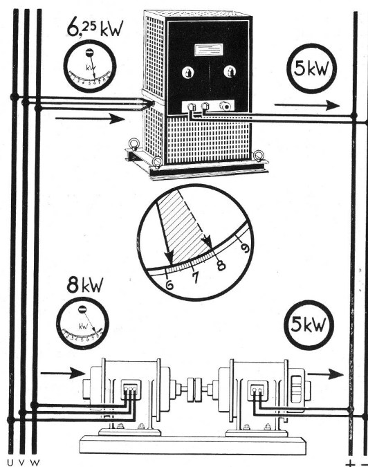
Schematische Darstellung der Wirtschaftlichkeit eines Kino-gleichrichters gegenüber der Umformergruppe.
