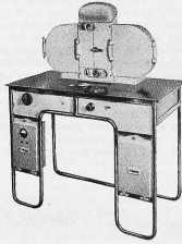
Tonkamera «Eurocord» Caméra d'enregistrement «Eurocord»
