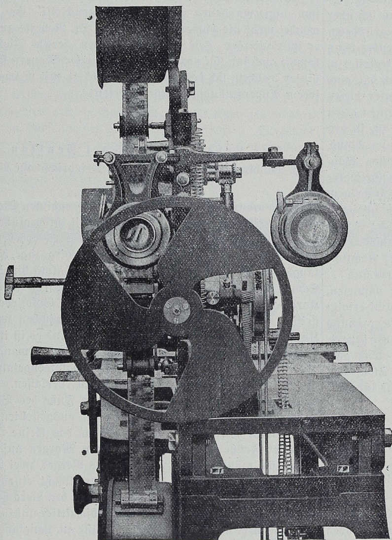
Neuester Original-Nitzsche-Apparat : Modell Nitzsche 1913.
