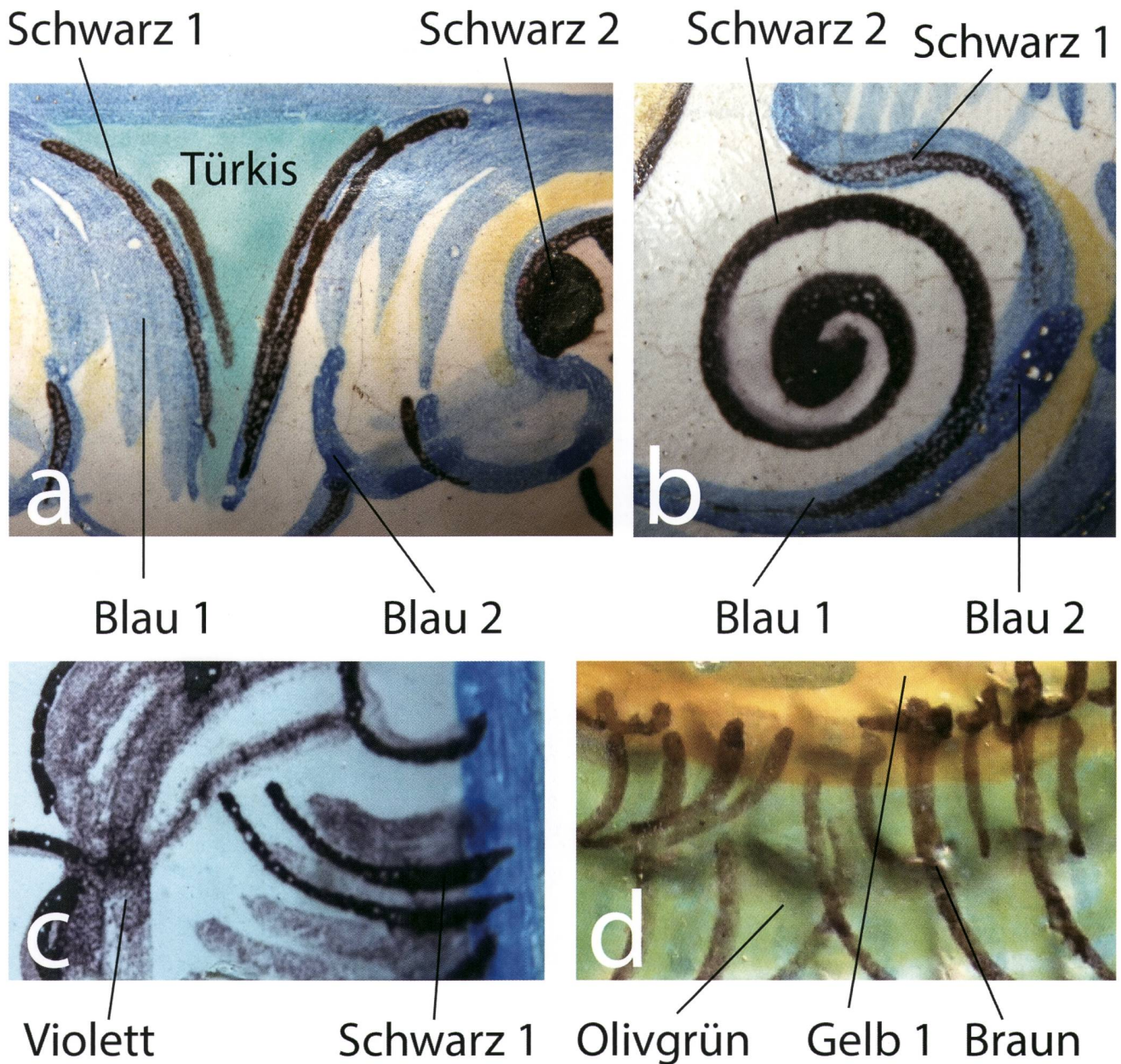
Abb. 11: Nahaufnahmen der Inglasurfarben und zeitliche Abfolge des Farbauftrags. (a) Ofe 25: Blau 1 / Türkis / Blau 2 / Schwarz 1 (blasig) und 2; (b) Ofe 26: Blau 1 / Hellgelb 1 / Blau 2 / Schwarz 2; (c) Ofe 24: Violett / Blau 2 / Schwarz 1; (d) Ofe 27: Olivgrün / Gelb 1 / Braun. Fotos M. Maggetti.
