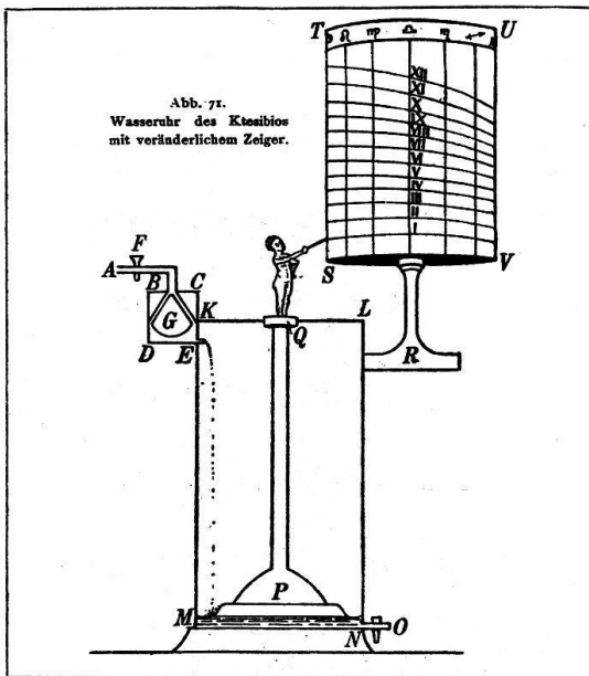
10 Wasseruhr-Grundmuster (nach Hermann Diels): «Das Wasser ergießt sich aus der durch den Hahn F abzuschließenden Leitung A in das Regulierbecken BCDE und tritt bei E durch eine feine Röhre in das Sammelbecken KLMN ein.» Für gleichmäßigen Wasserdruck sorgt der Pfropfen G, der bei übermäßiger Wasserzufuhr sich hebt und den Zufluß stoppt. «So spritzt in feinem Strahle das Wasser in das Hauptbecken KLMO. Dort hebt es den Schwimmer P, auf dem oben ein Figürchen angebracht ist, das mit einer Rute die zwölf Stunden anzeigt. Sie sind in Horizontalkurven auf dem drehbaren Zylinder STUV angebracht» und verschieden «lang», je nach der, durch die Sternzeichen über den Senkrechten, markierten Jahreszeit. Antike Uhren erforderten genaue Wartung. Bei unserem Typ war täglich der Behälter zu leeren und das «Zifferblatt» um «einen Tag» weiterzudrehen (S. 205–208).
