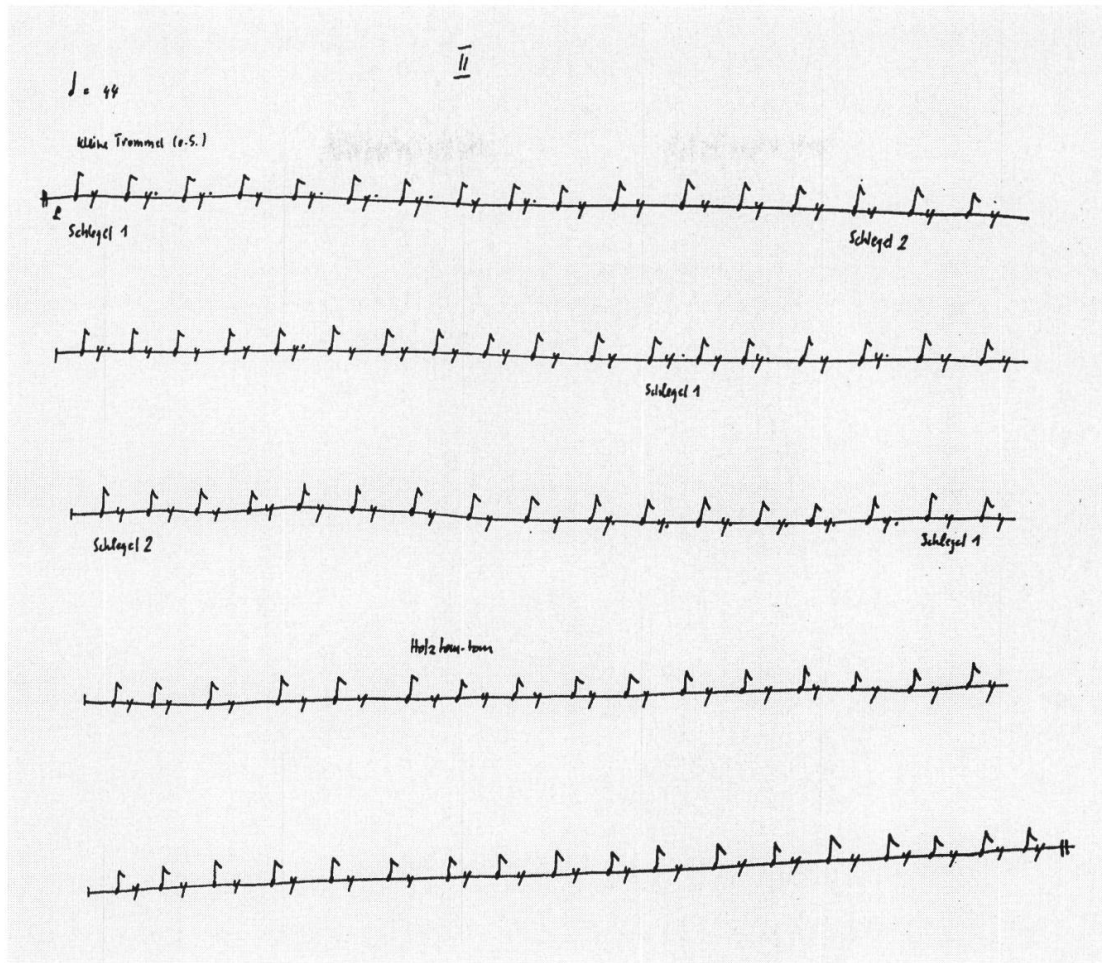
Notenbeispiel 6
