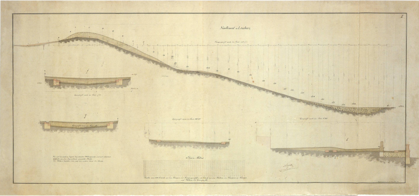
Plan Nr. 1 Längenprofil I, A. Negrelli (1839)
