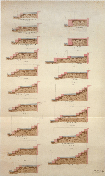
Plan Nr. 4 Querschnitt, A.H. Hünerwadel (1856)
