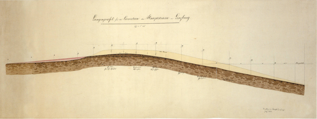
Plan Nr. 5 Längenprofil, Baumeister Wolf (1856)
