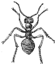
Fig. 7. Ouvrières du Formica rufa vues de face et de profil et très grossies.
