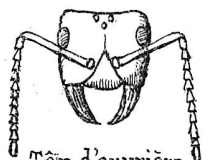
Tête d'ouvrière ( Polyergus rufescens Latr.) très grossie.
