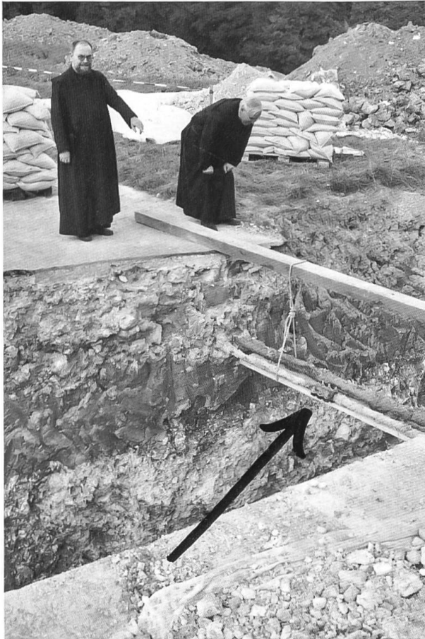
P. Norbert und P. Ignaz inspizieren die Baustelle beim «Wilerrank». Befriedigt stellen sie fest, dass die Leitung für das sog. Klosterwasser (Pfeil) intakt geblieben ist; sie wird jetzt von norwegischem Erdgas unterquert.
