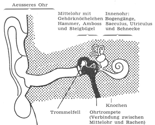
Abb. 36: Die Teile des Ohres (Uebersicht)
