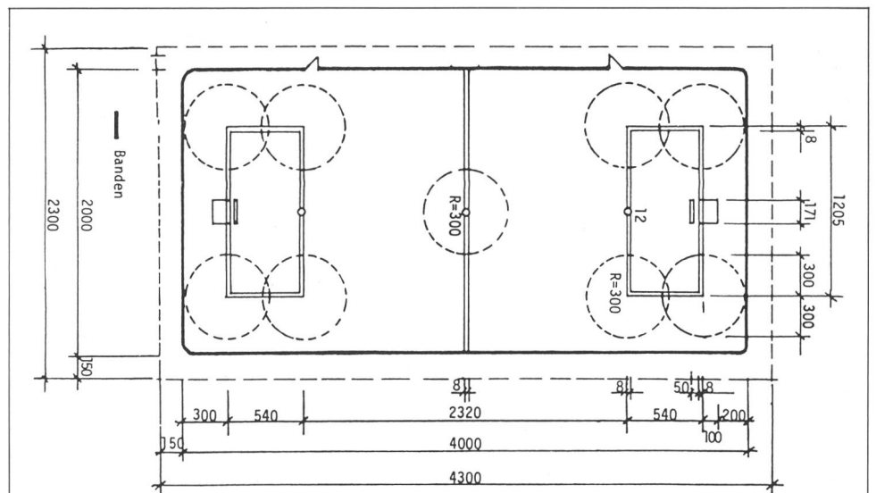
Hockey su pista. Dimensioni del campo da gioco 34 x 17 fino a 40 x 20 m (misura raccomandata). Zone e distanze di sicurezza raccomandate: 1,50 m. Indicazioni: pavimentazione di cemento. Reti di protezione dietro le porte alte almeno 2 m.
