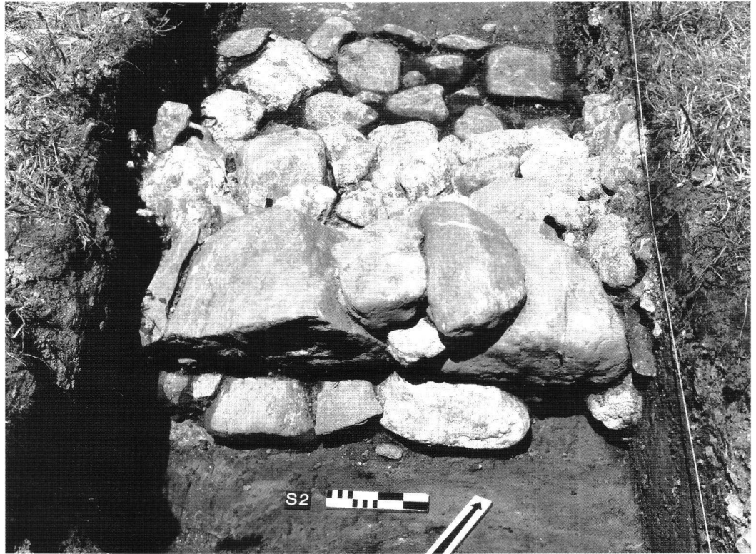
Abb. 14: Letzi Rothenturm 1999. Schnitt S2. Freigelegte Abbruchkrone der Letzimauer. Der feindseitige Mauermantel (hinten im Bild) ist bis auf das Fundament hinab abgebrochen. Vor der untersten Steinlage des freundseitigen Mauermantels ist der gut 10 cm vorspringende Fundamentabsatz gut zu sehen. Blick von Südsüdosten.
