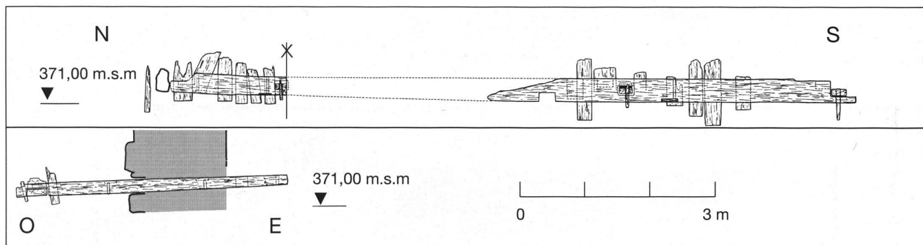
11: Vue de face et coupe de la fondation de la tour.
