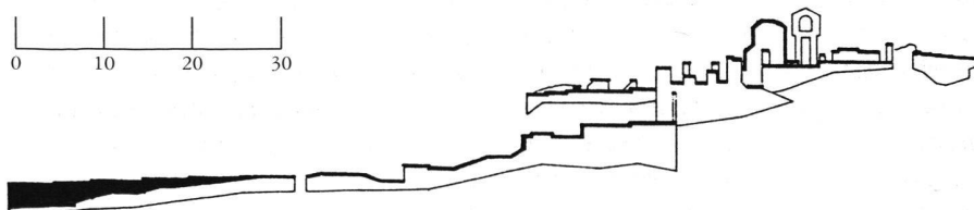
12: Profilo del progetto – Längsschnitt durch die Burg mit den geplanten Veränderungen an der Südseite (links).
