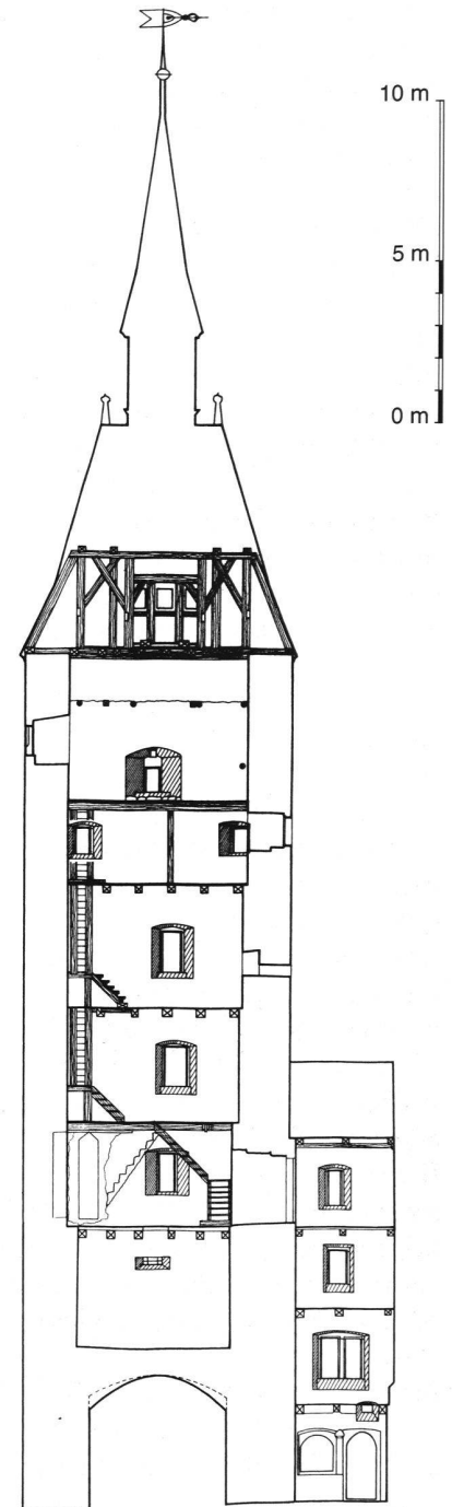
2: Schnitt durch den Spittelurm nach Westen. M. 1:250.
