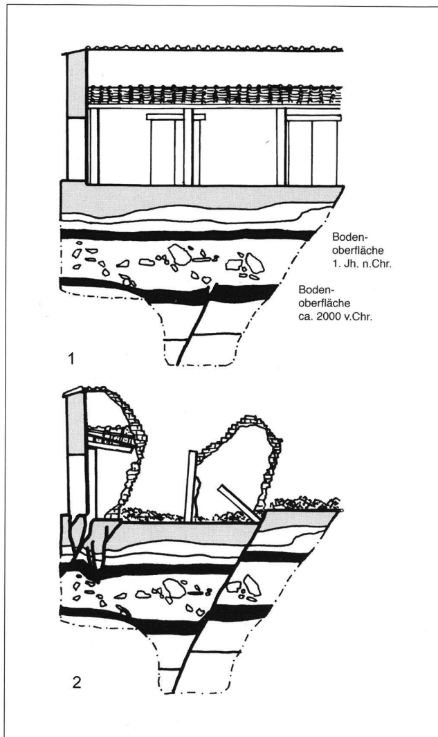
11: Egnatium (I). 1. Vertikale Verschiebung von Erdschichten im Untergrund beim Erdbeben zwischen 2581 und 2197 v.Chr. Danach Ablagerung von Flusssedimenten. 2. Zerstörung des römischen Gutshofs beim Erdbeben Mitte des 3. Jh. n.Chr.
