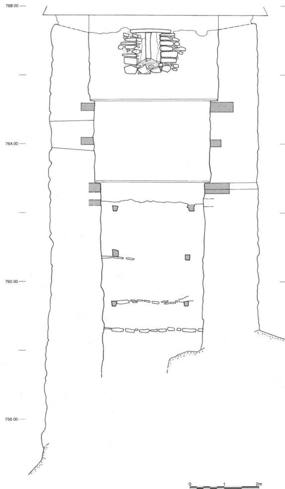
6: Innenwand Nord mit Schartenfenster im 2. Obergeschoss und sechs Gerüstbalkenlöchern im Sockelgeschoss. Das Loch rechts oben wurde nachträglich zugemauert.
