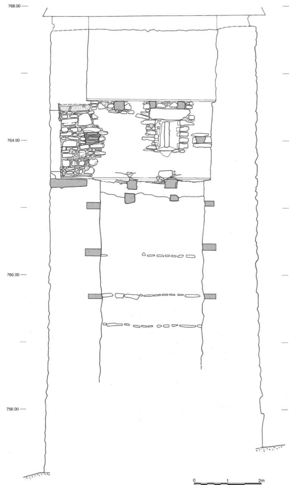
7: Innenwand West mit Schnitt durch den Hocheingang, Lichtnische und Schartenfester im 1. Obergeschoss. Die zwei Balken des Fussbodens im 1. Obergeschoss wurden vermutlich im Zuge einer Bauplanänderung etwas nach oben versetzt.
