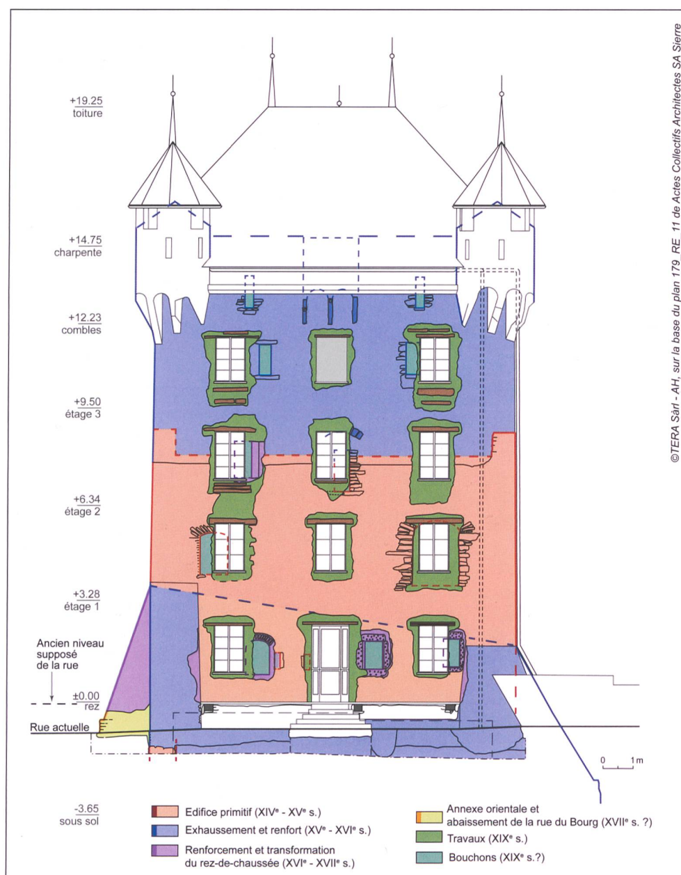
7: Sierre VS, tour des Vidomnes. Relevé archéologique de la façade ouest.
