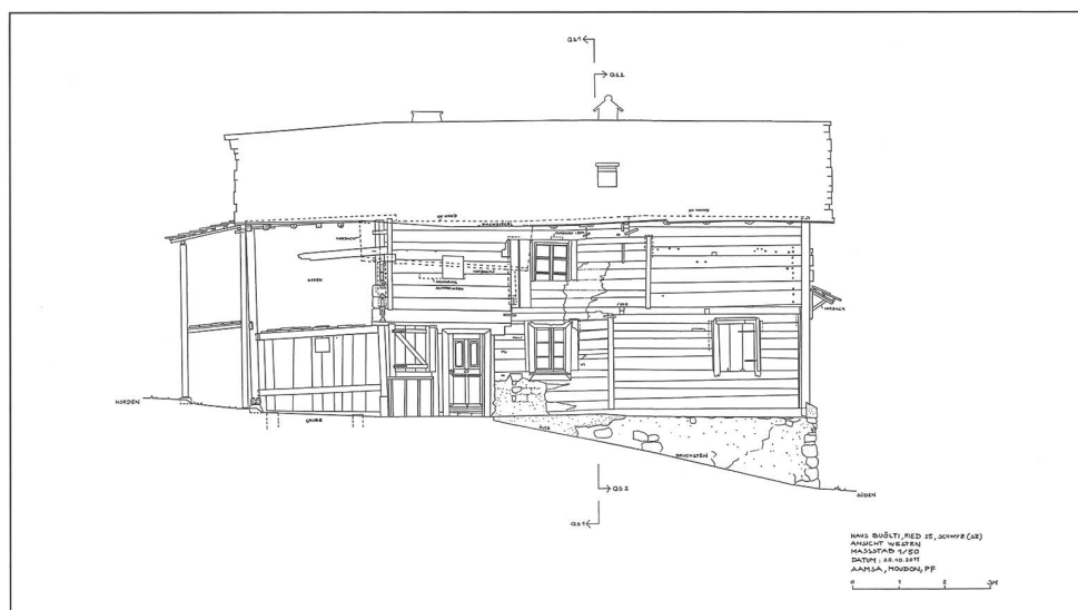
8: Schwyz SZ, Haus Büölts. Westliche Hausfassade mit Sockelgeschoss unter dem Vorderhaus und Auflage des Hinterhauses auf dem Hang.
