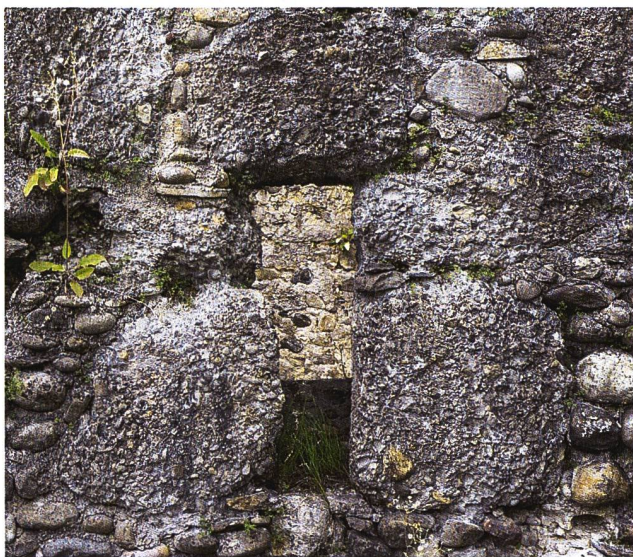
45: Häggenschwil SG, Ruine Alt Ramschwag. Hochrechteckiges Schartenfenster 11.2, äusseres Gewände, ausschliesslich aus Nagelfluhquaden zusammengesetzt. Aufnahme 2022, von Nordosten.
