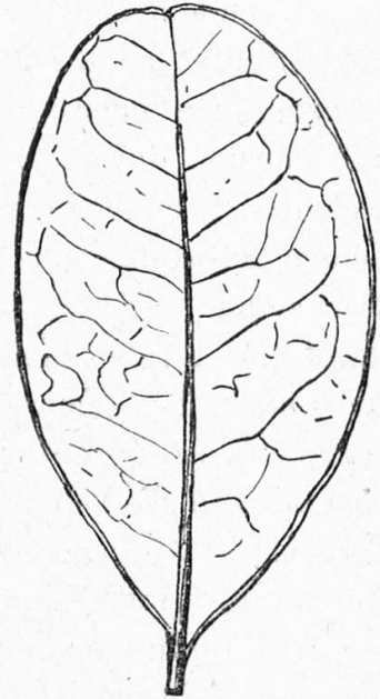
Fig. 27. Ilex caaguazuensis . (Grandeur naturelle.)
