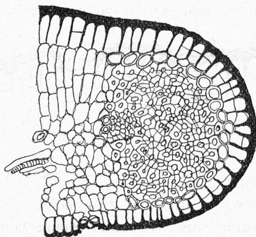
Fig. 39. Faisceau fibreux de la marge de la feuille.
