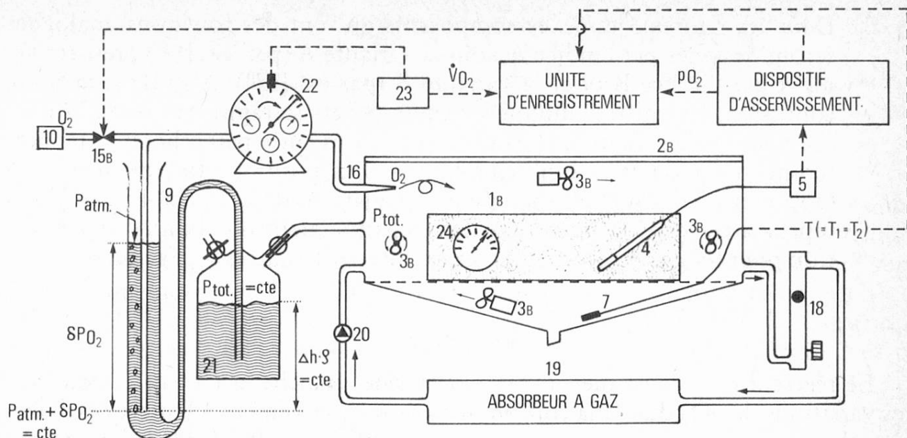
Fig. 4. Détail de l'analyseur proposé pour les macromesures (variante B)
