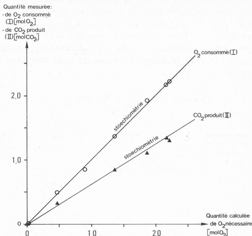
Fig. 5. Vérification expérimentale du fonctionnement du dispositif proposé (variante B pour macromesures) en utilisant la combustion complète du butane comme réaction d'oxydation stoéchiométrique modèle
