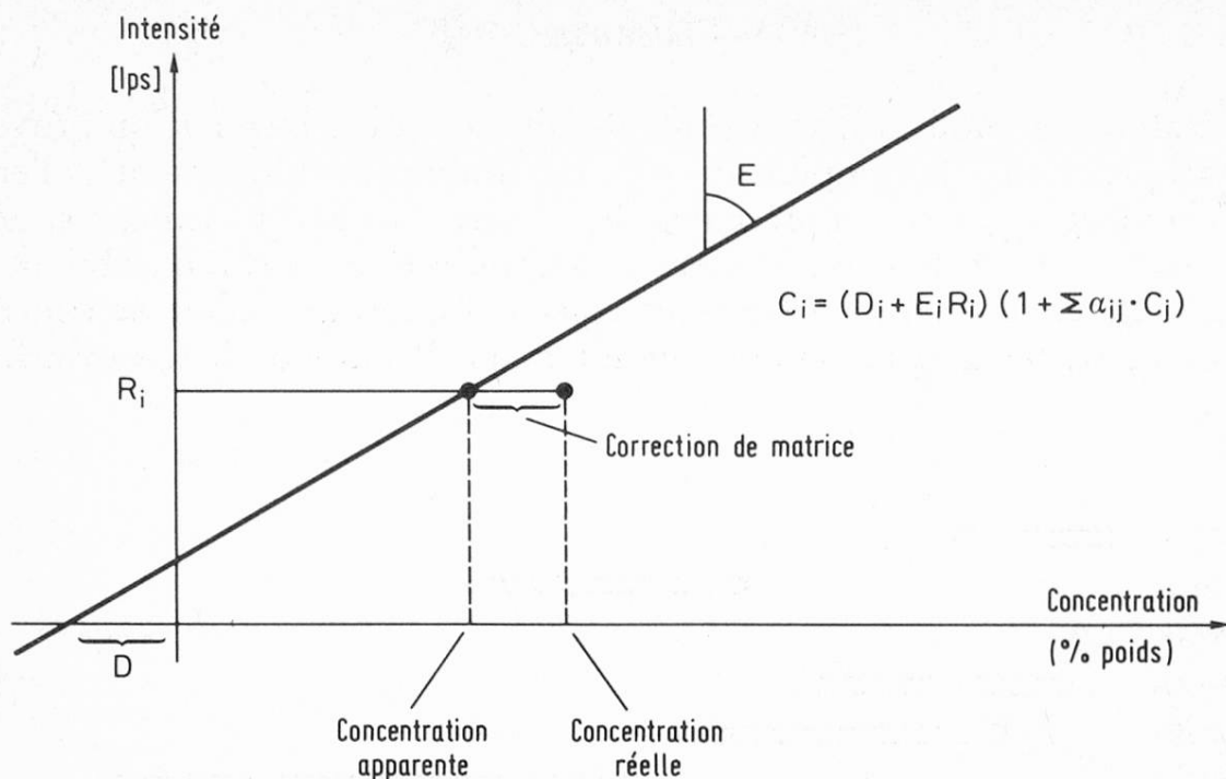
Fig. 2. Droite d'étalonnage
