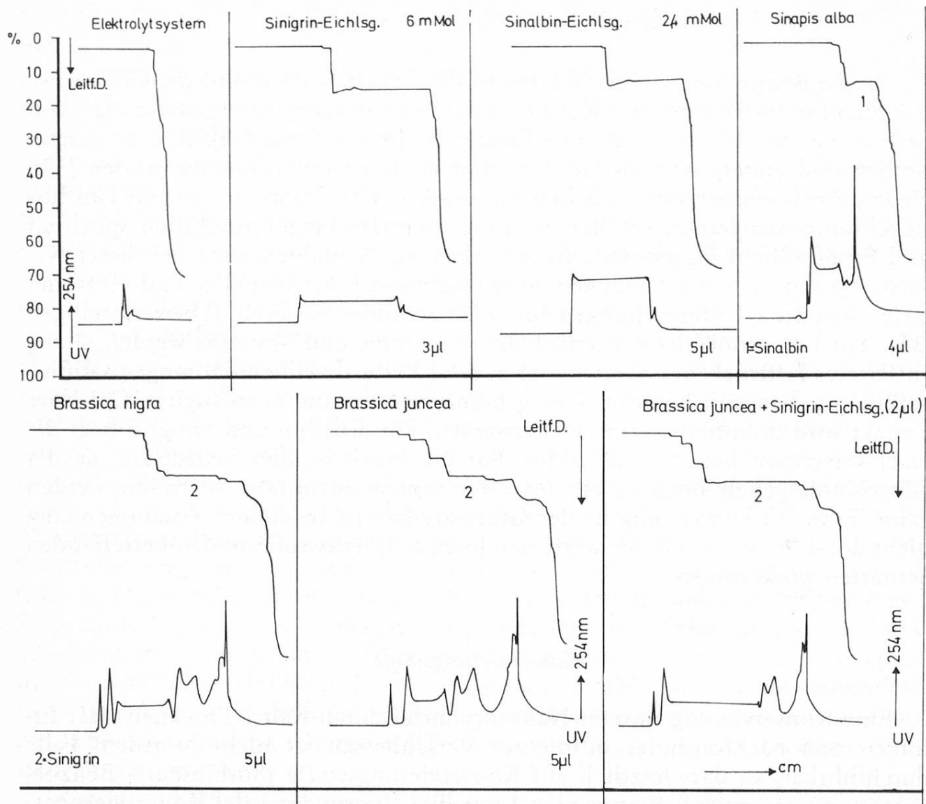
Abb. 1. Isotachophoretische Bestimmung von Sinalbin und Sinigrin in Samenextrakten von drei Senfarten sowie UV- und Leitfähigkeitsdiagramme des Elektrolytsystems und der Reinsubstanzen. (Entnommen aus: «Z. Acker- u. Pflanzenbau» 150, 353 [1981]. Mit Genehmigung des Verlages.)
