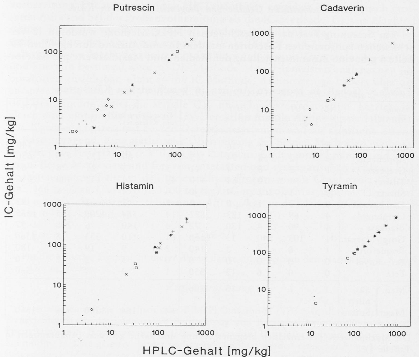
Abb. 3. Vergleich der HPLC- und der IC-Bestimmung der biogenen Amine Putrescin, Cadaverin, Histamin und Tyramin
