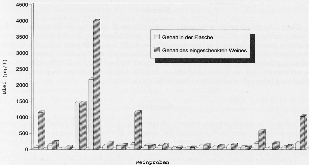
Abb. 9. Einfluss der Blei-Zinn-Folien auf den Bleigehalt im Wein
