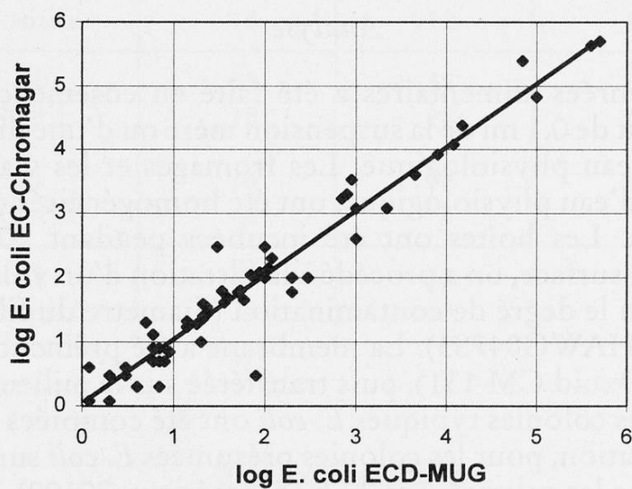
Fig. 2. Comparaison par régression linéaire du milieu de culture ECD-MUG (méthode de référence) au milieu chromogène EC-Chromagar
