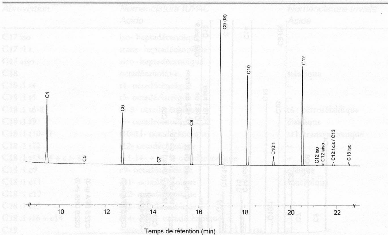
Figure 2 Chromatogramme partiel des acides gras C4 à C13 iso
