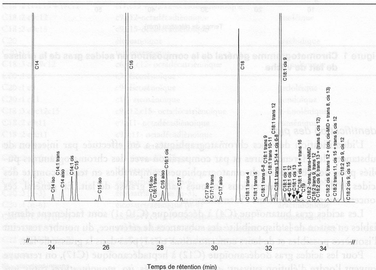
Figure 3 Chromatogramme partiel des acides gras C14 à C18 :2 cis 9, cis 15
