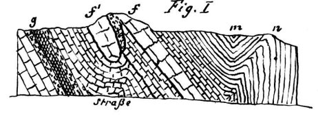
Fig. I II. Locale Stauchungen im oberem Jura. Dessenbergstrasse
