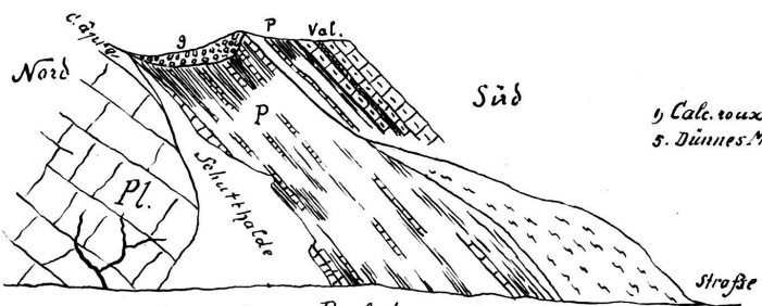
Profil durch das Purbeck westl. von Tüscherg.
