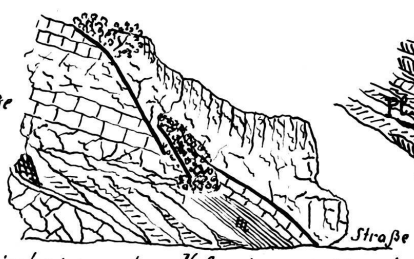
Hornische im unteren Valangien, westl. von Tüscherg. m = Mergel mit Fossilien. a = Dislocation breccie
