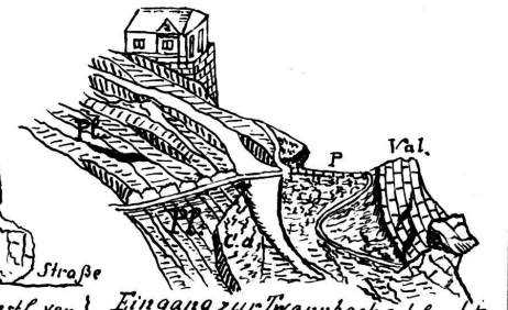
Eingang zur Trambachschlucht C.a. = Calcaire à pure.
