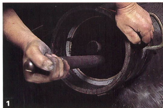
1 Pilonnage du sable de Paris autour du modèle.
