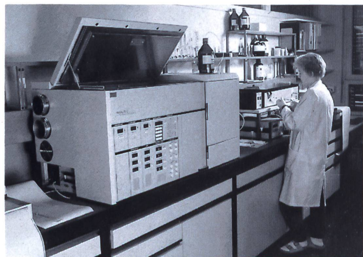
Esame nel laboratorio chimico per accertare la biodegradabilità di sostanze nocive immerse nell'acqua.
