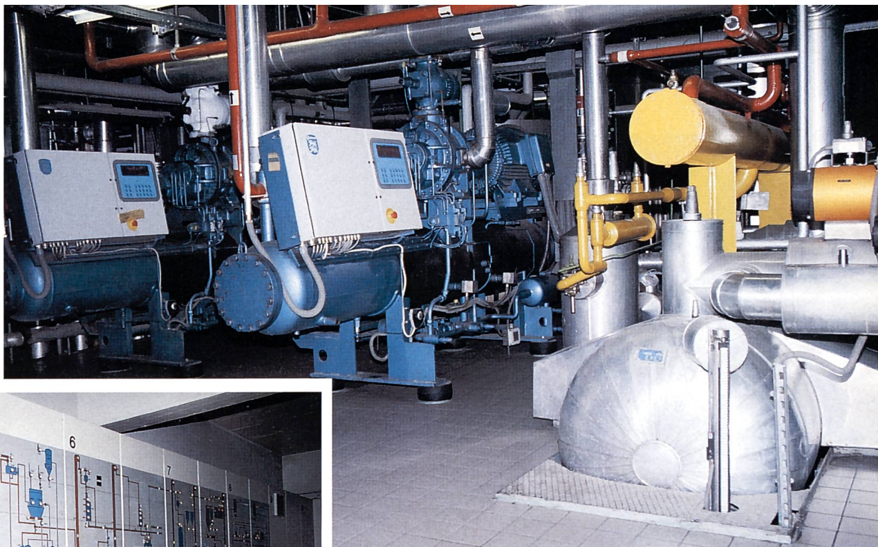
Compressori frigoriferi di deodorazione
