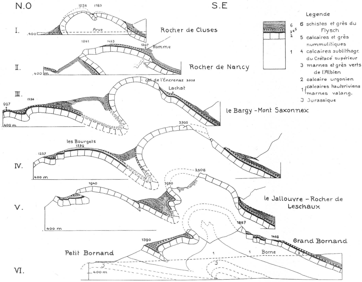
Profils de la chaîne des Vergy - Rocher de Cluses (H te Savoie)
