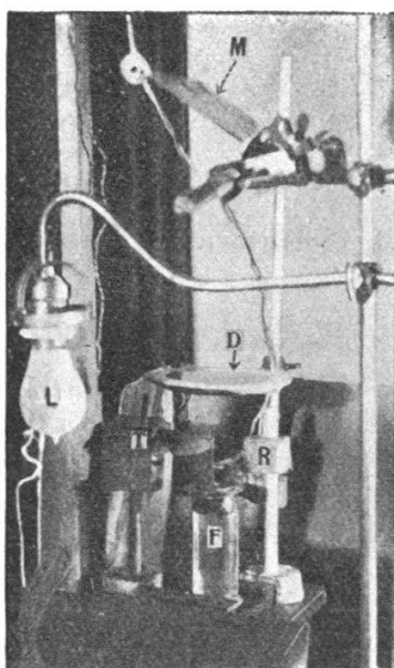
FIG. 16. — F, feuille disposée pour l'observation ; R, résistance de chauffage ; T, thermomètre ; D, disque gradué ; M, miroir ; L, lampe auxiliaire.
