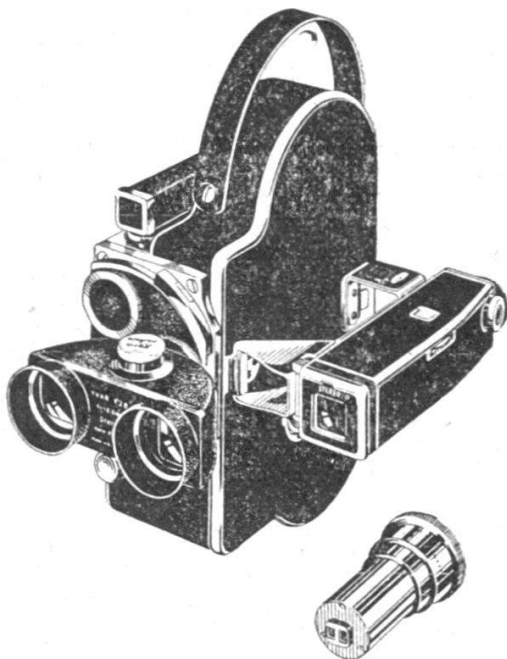
Caméra H 16 munie de l'accessoire stéréo Kern-Paillard.
