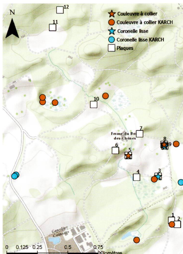
Figure 4. Carte du Bois de Chênes et observations des serpents (en orange: couleuvre à collier; en bleu: coronelle lisse). Les données disponibles avant le suivi (fournies par le karch) sont représentées par des points, les données récoltées pendant le suivi par des étoiles.
