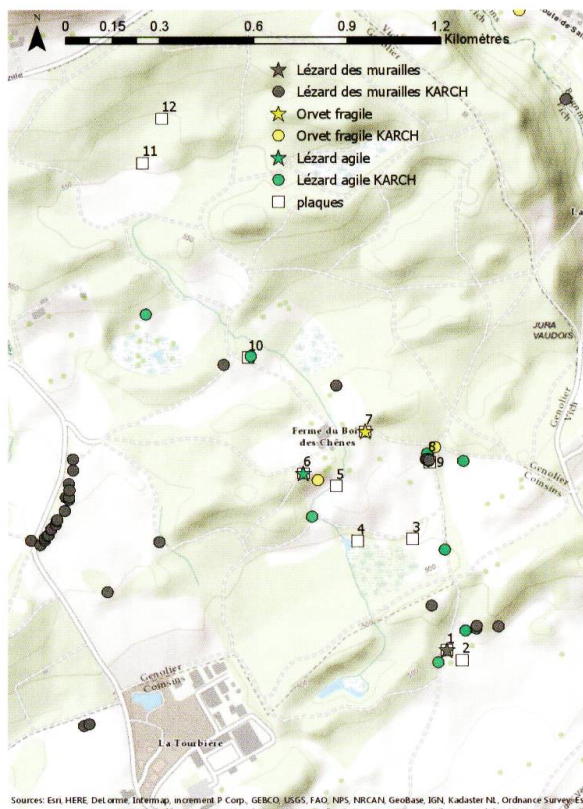
Figure 5. Carte du Bois de Chênes et observations des lézards (en gris: léopard des murailles; en jaune: orvet fragile; en vert: léopard agile). Les données disponibles avant le suivi (fournies par le karch) sont représentées par des points, les données récoltées pendant le suivi par des étoiles.
