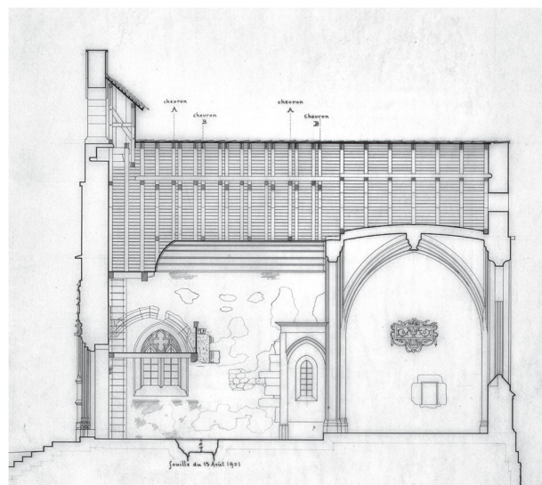
4 Relevé de l'église de Treytorrens par Paul Nicali, coupe longitudinale, sans date (ACV, AMH, B 320b, 1, B 2864).
