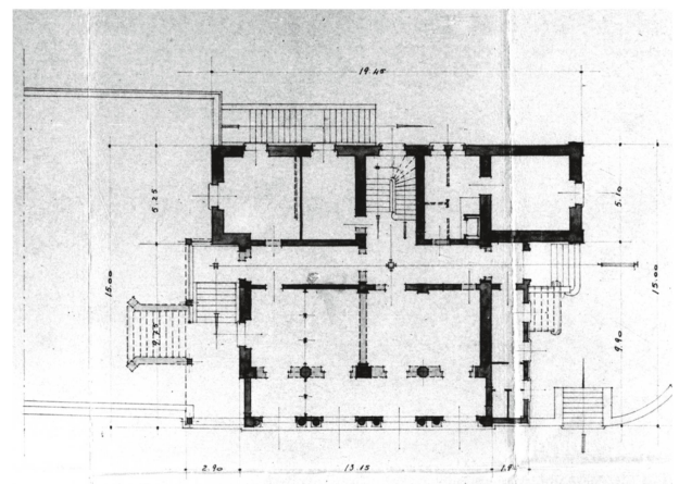
6 Plan du rez-de-chaussée, René Bonnard et Félix Damia architectes, 17 août 1933. En grisé, éléments à démolir (AVL, dossier de mise à l'enquête publique).
