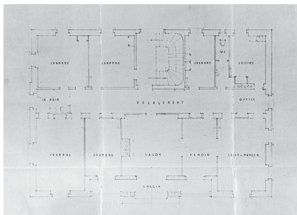
8 Plan de l'état initial de la villa Faucigny à l'avenue d'Évian 4, réalisé en 1936 en vue de transformations. Ici, il s'agit du troisième étage, qui met en évidence la présence de la loggia, inexistante aux étages inférieurs (AVL, police des constructions).
