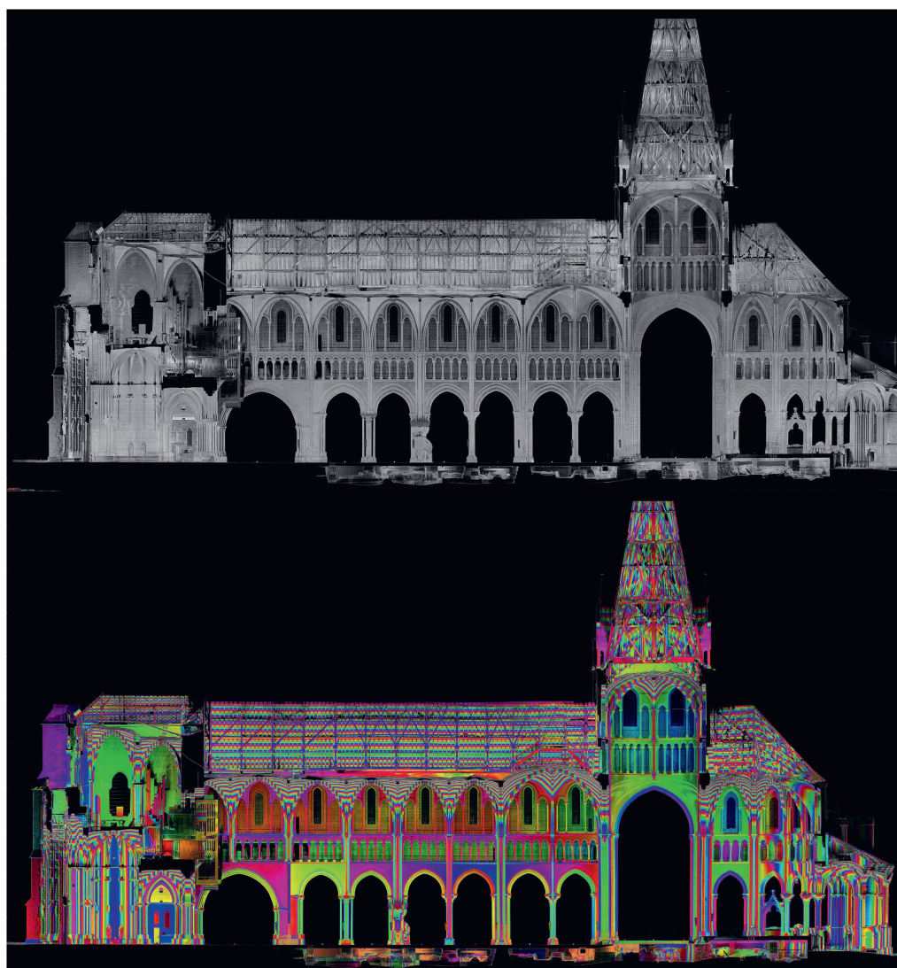
4 Le nuage de points peut être coupé et projeté selon n'importe quel plan de l'espace; ici, la coupe longitudinale de la cathédrale avec, en haut, l'image en intensité de lumière laser et, en bas, l'image colorisée par profondeur des pixels par rapport au plan de coupe par bandes d'un mètre.
