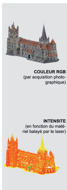
Nuage de points 3D de la morphologie de la cathédrale
